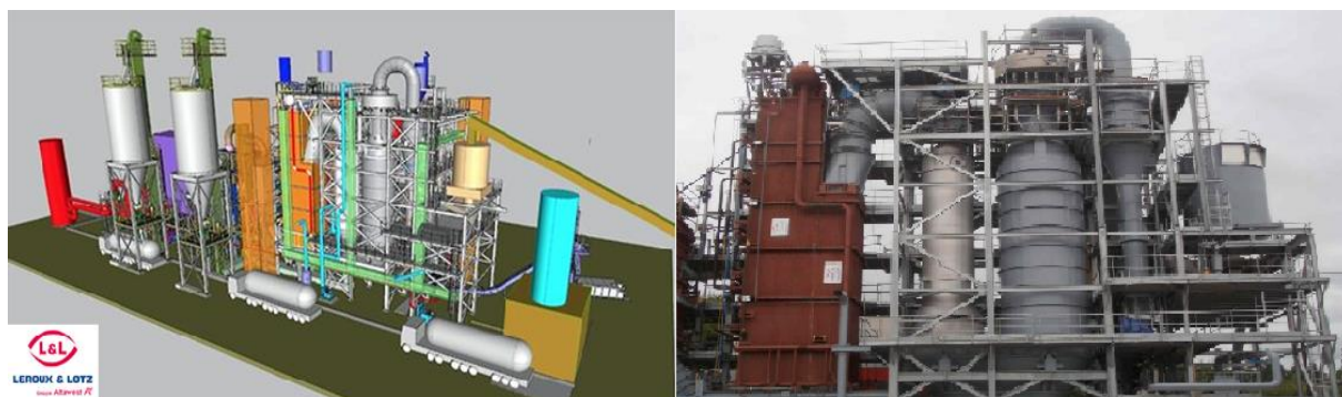
Figure 83 The Synnov Déchets Viller-sur-Montrond plant 448
